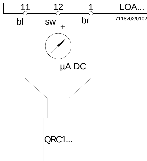
Abb. 43: Mess-Schaltung zur Fühlerstrommessung
