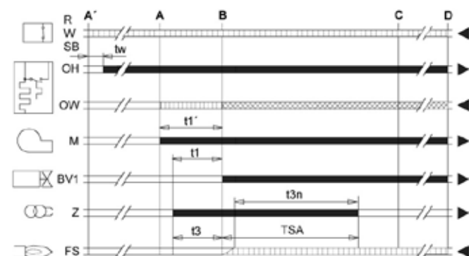
Abb. 28: Programmablauf LMO 14.155
