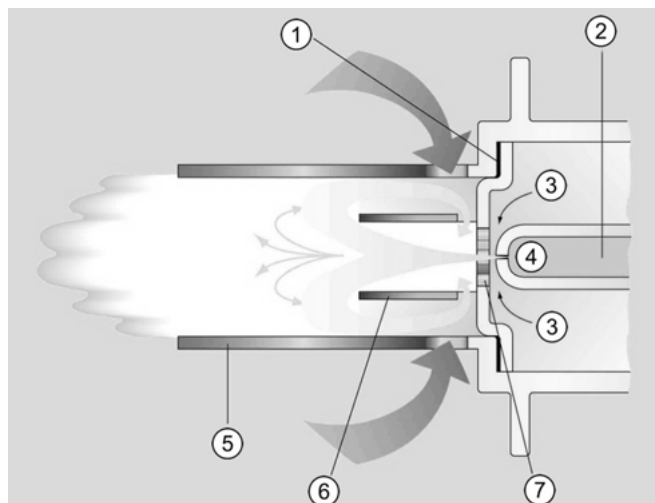
Abb. 48: Verbrennungsablauf Raketenbrenne®
