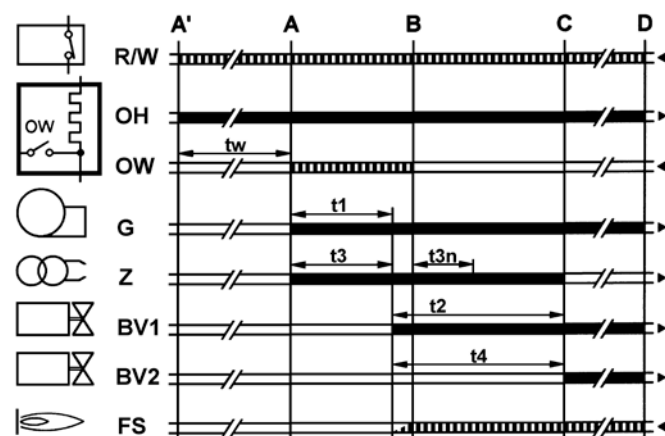
Abb. 29: Programmablauf LMO 44.255
