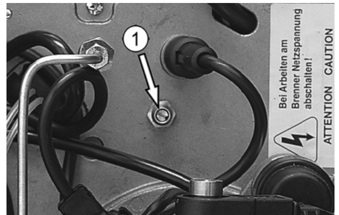
Abb. 24: Messnippel ① zur Prüfung der Gebläsepressure
