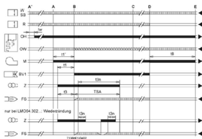
Abb. 30: Programmablauf LMO 64.301
