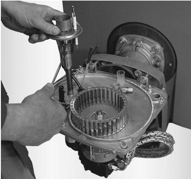
Abb. 35: Demontage Mischsystem
