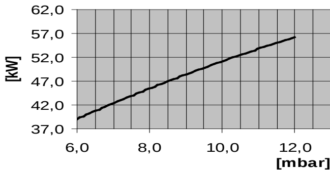
Abb. 21: Leistungsdigramm RE 1.50 H
